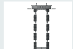
Basismodell mit 4 Paar Aufsätzen 191 - 199 mm
